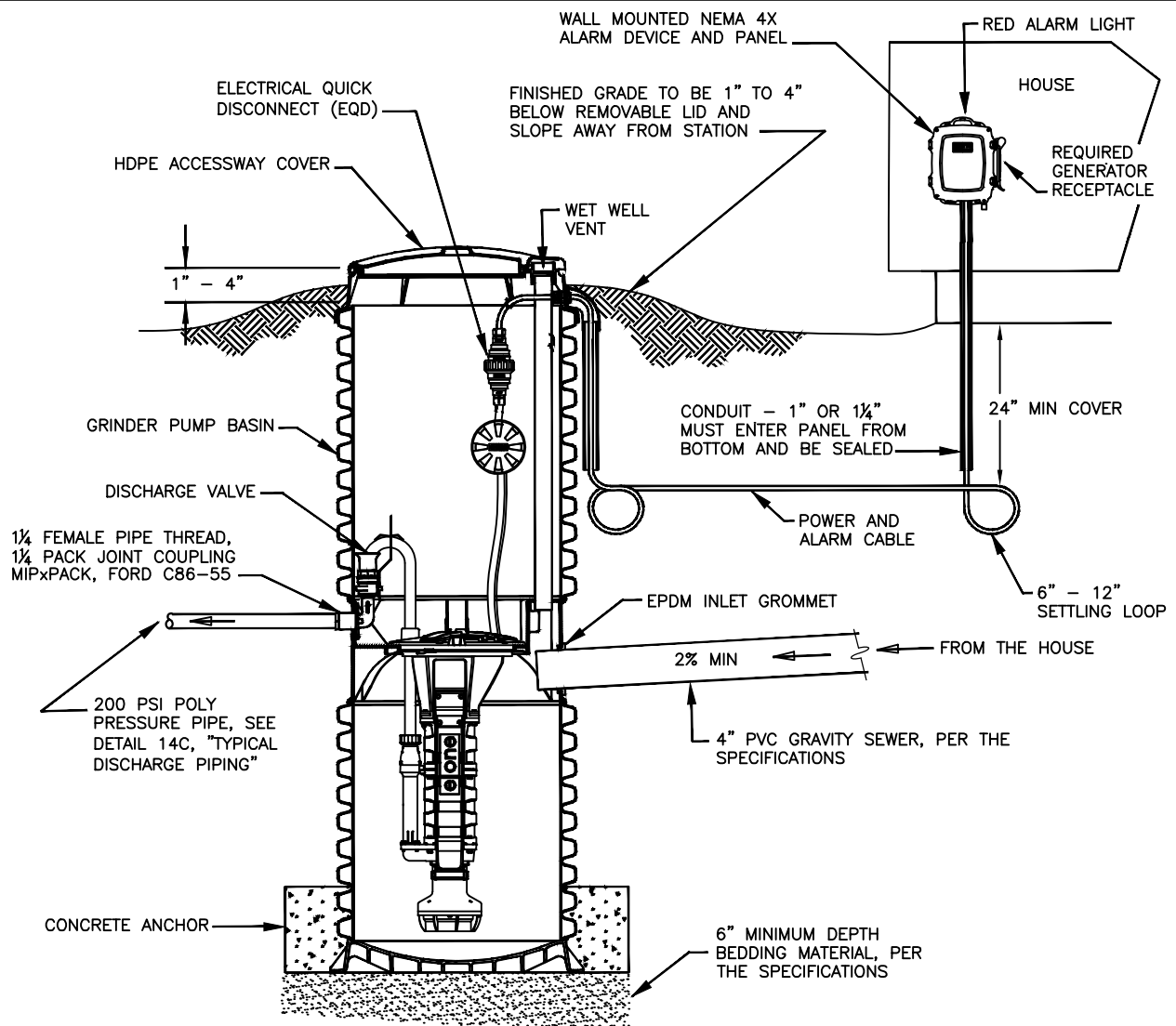
ELEVATION
