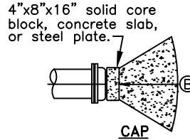
CAP
